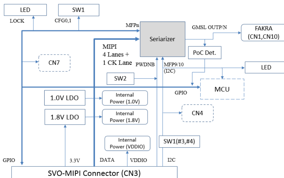
ブロック図
