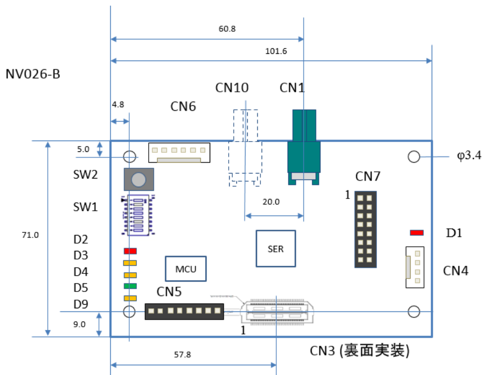
主要コネクタ配置図
